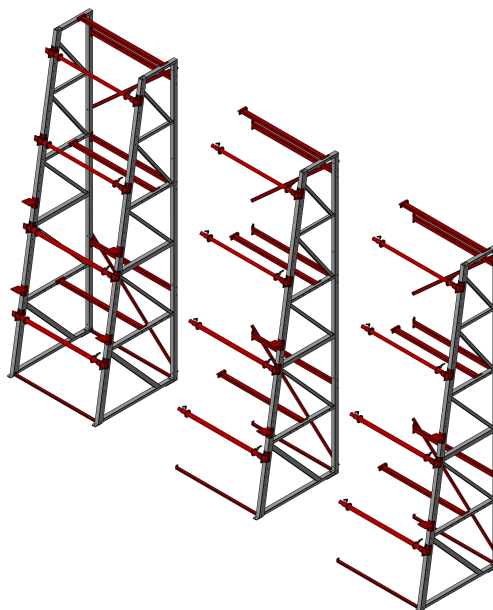
Рис. 5 Стеллажный ряд
