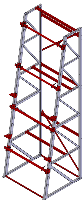
Рис. 1 Основной пролёт
