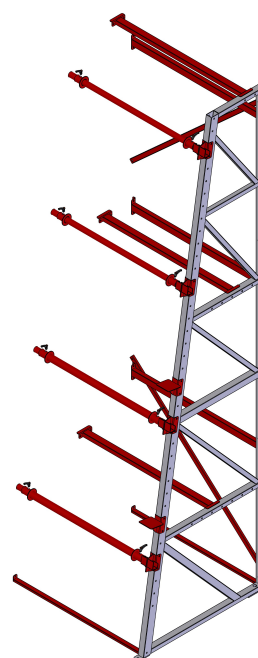
Рис. 2 Дополнительный пролёт
