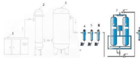
Адсорбционные осушители
