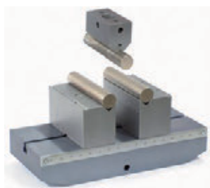
Устройство на трехточечный изгиб
