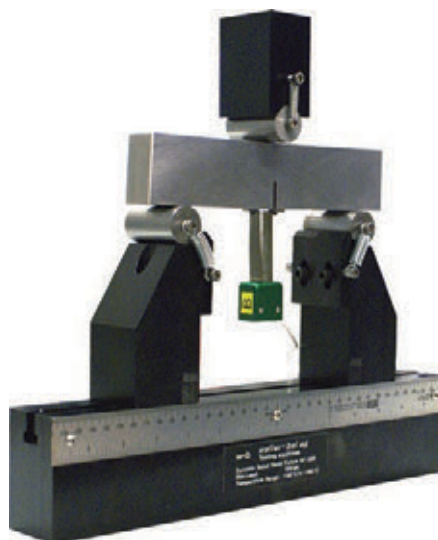
Устройство для испытаний образцов в виде балок (SEB) по схеме трехточечного изгиба
